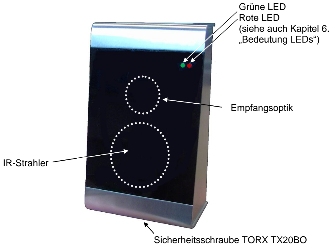
Abbildung 3: Übersicht Komponenten Weitbereichsleser APX2
