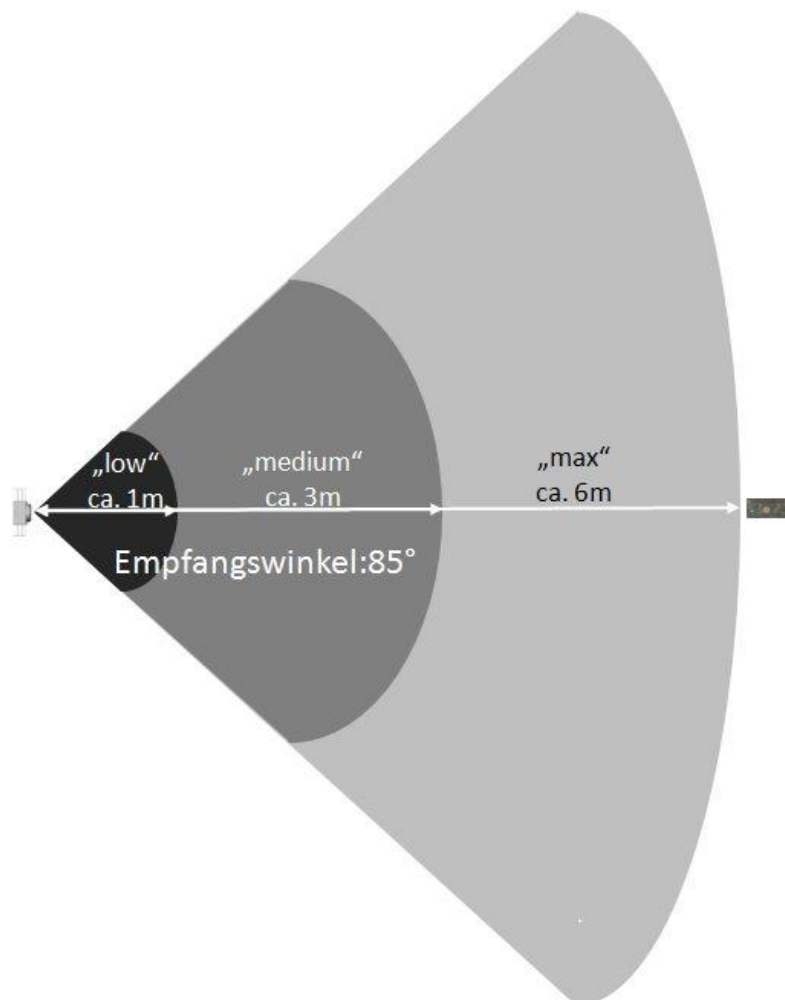
Abbildung 11: Zusammenhang Empfindlichkeit und Lesereichweite
