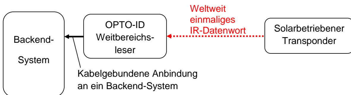
Abbildung 1: Blockschaltbild Funktionsprinzip OPTO-ID
