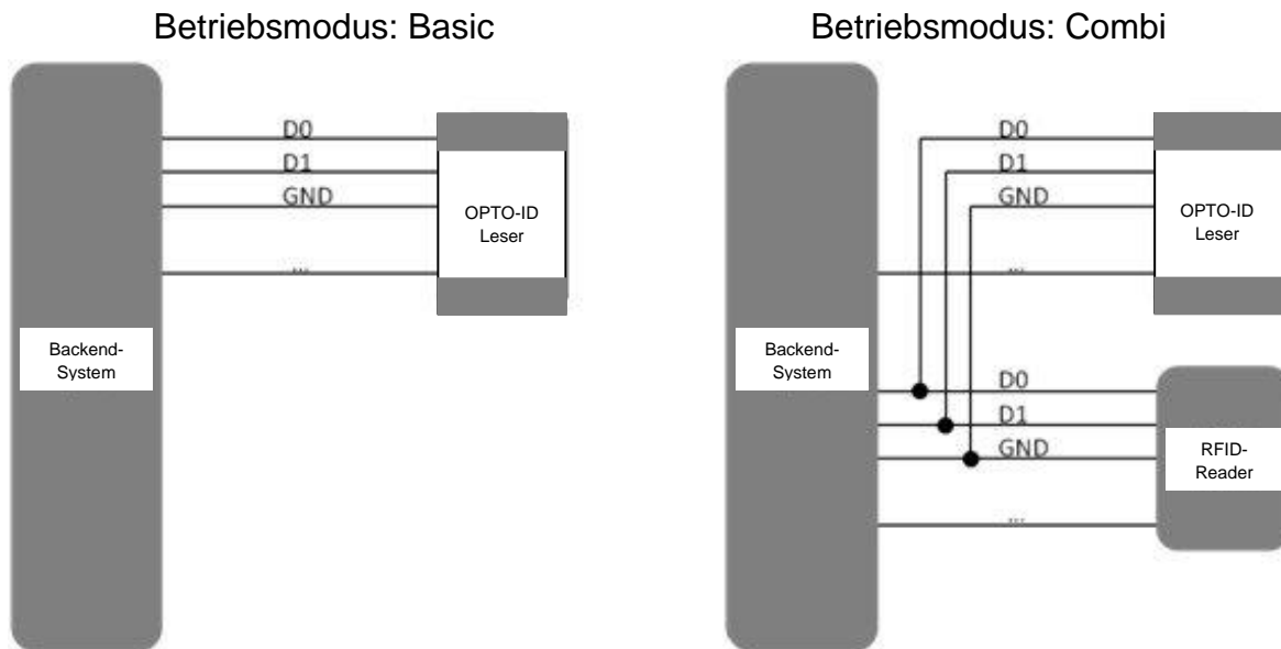
Abbildung 6: Anschluss des P-ID Lesers für verschiedene Betriebsmodi (links: Basic / rechts: Combi)
