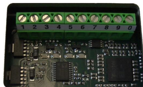
Abbildung 7: Anschlussklemme P-ID Leser
